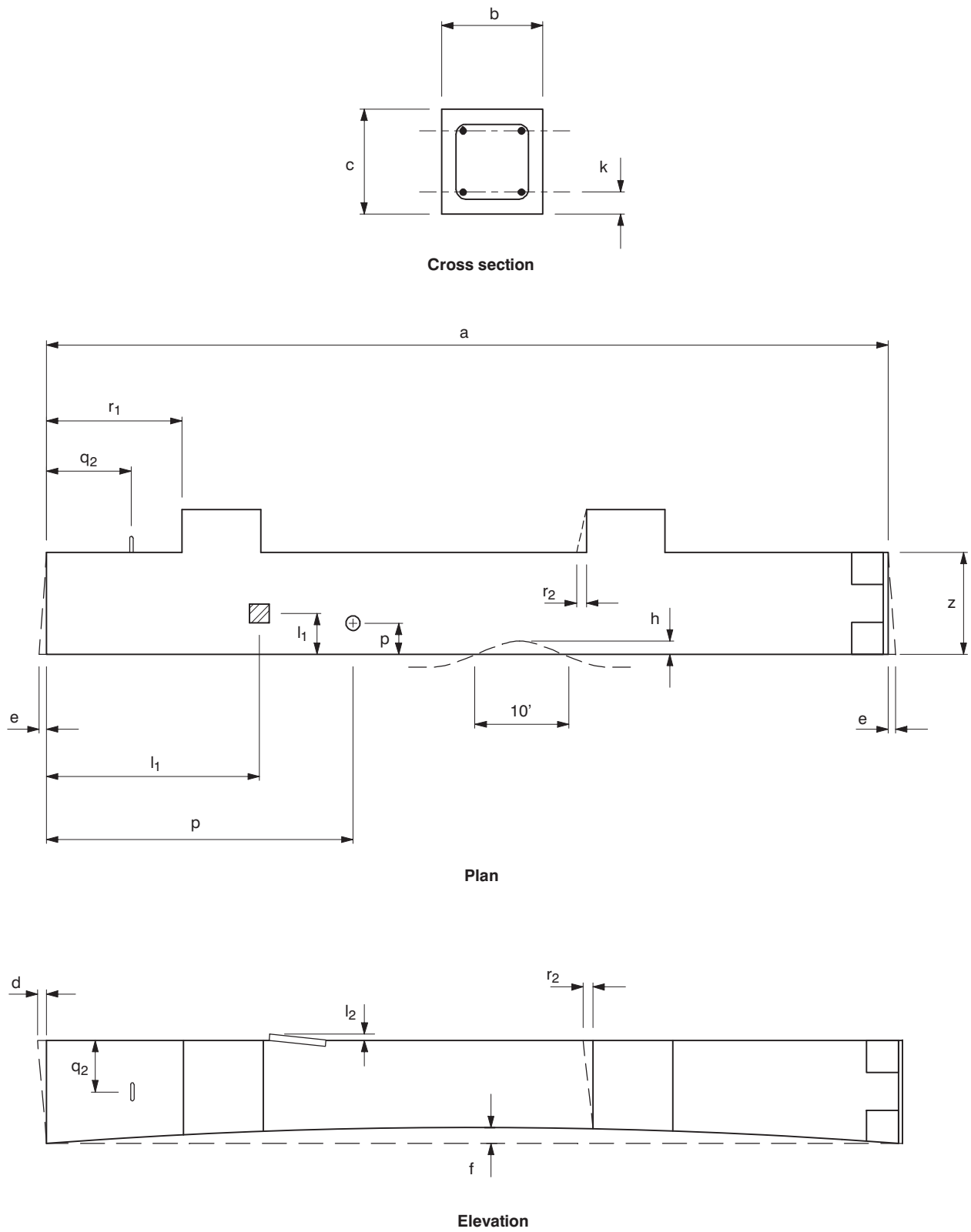
Fig. 10.8.1 Columns
