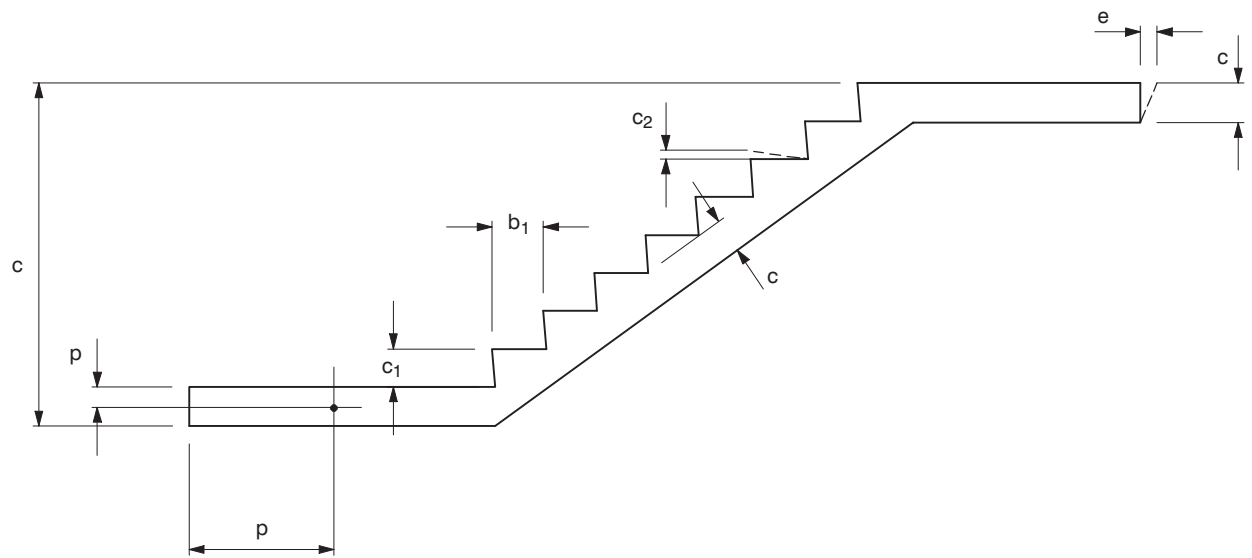
Elevation
