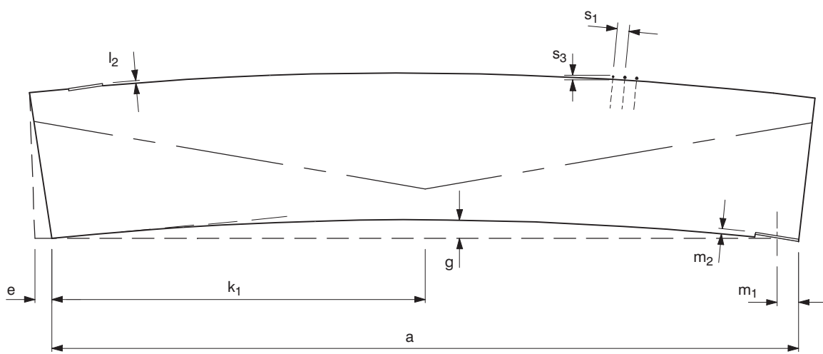
Elevation
